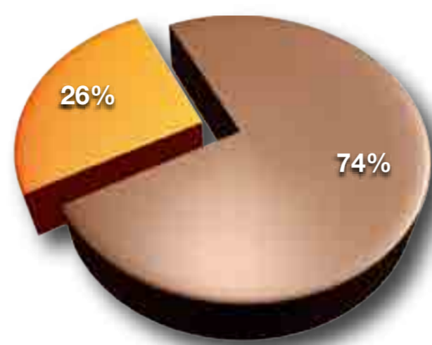
MONTE CANONI 2008
